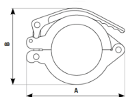
GIUNTO COMPLETO A LEVA
